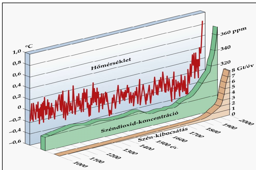
1.2. ábra – A hőmérséklet, a CO 2 koncentráció és a CO 2 kibocsátás alakulása az elmúlt 1000 évben
