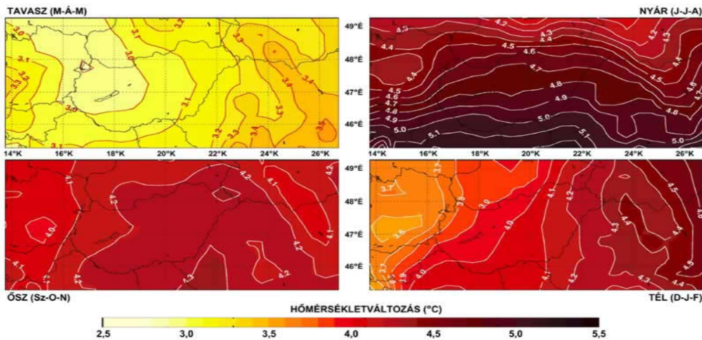
1.4 ábra - Évszakai hőmérsékletváltozás (°C) a Kárpát-medence térségére a PRUDENCE projektben alkalmazott európai regionális (50 km-es rácsfelbontású) éghajlati modell eredményei alapján a 2071–2100 időszakra
